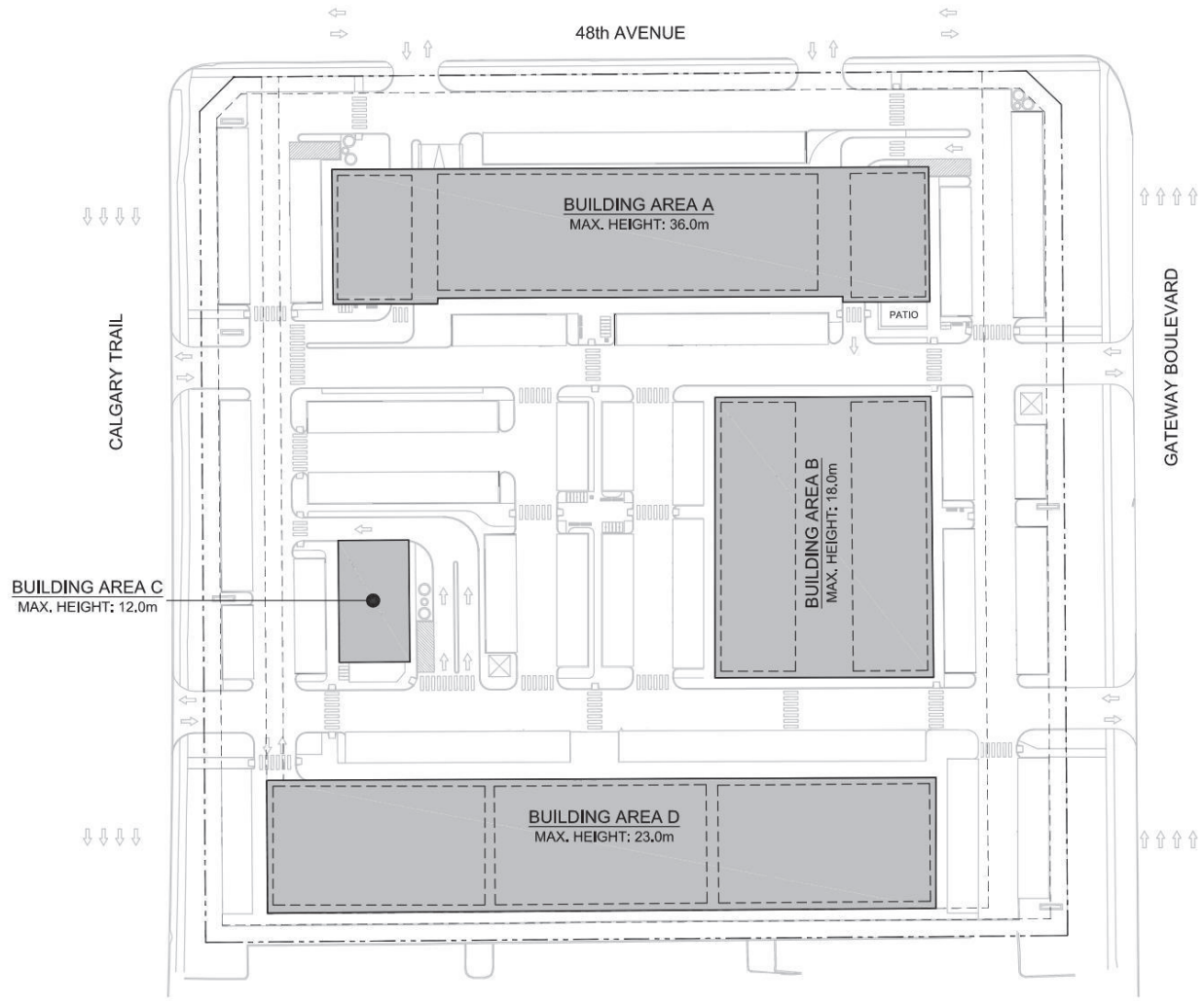
Site Plan 4710 - Gateway Boulevard NW
